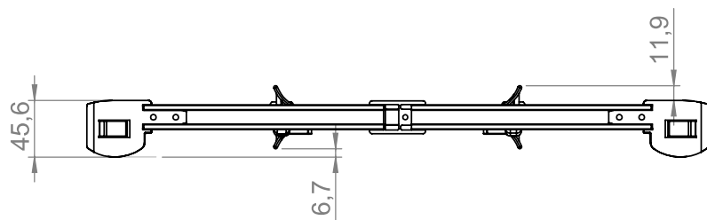
SEZIONE ORIZZONTALE
